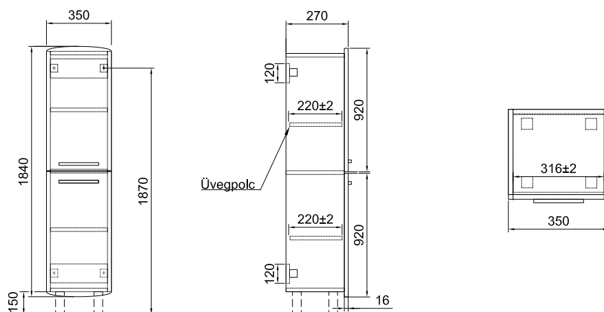
Tükrosszekrény világtás nélkül A498 60 xx
