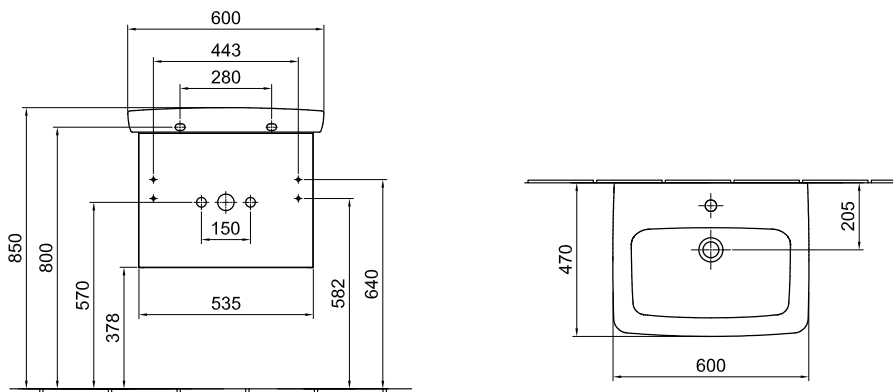
Mosdószekrény B537 00 xx
