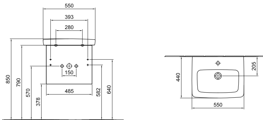
Mosdószekrény B537 00 xx
