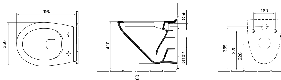
Mélyöblítésű fal-WC 7048 R0 xx
